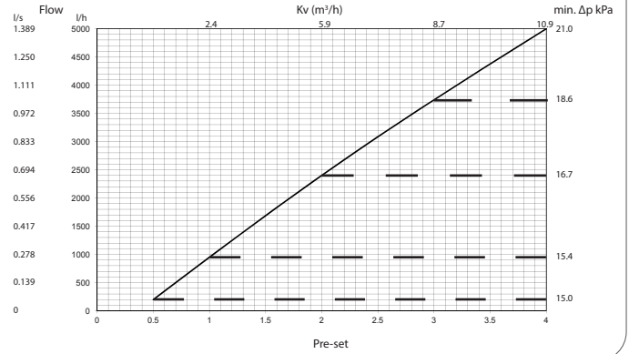
SIGMA Compact DN32
